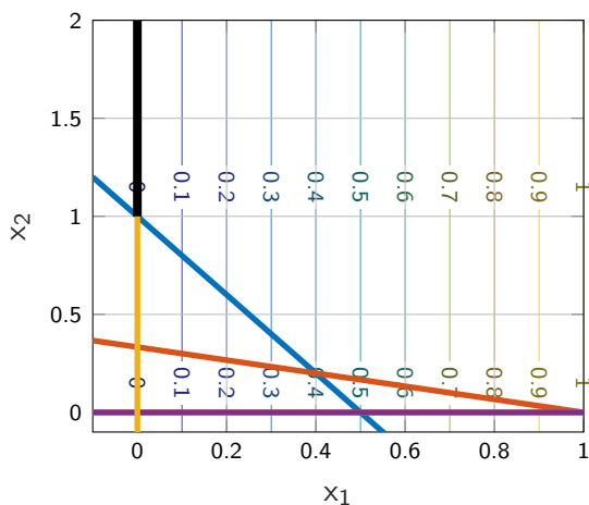
Abbildung 2: Höhenlinien und optimale Punkte für die verschiedenen Kostenfunktionen.
