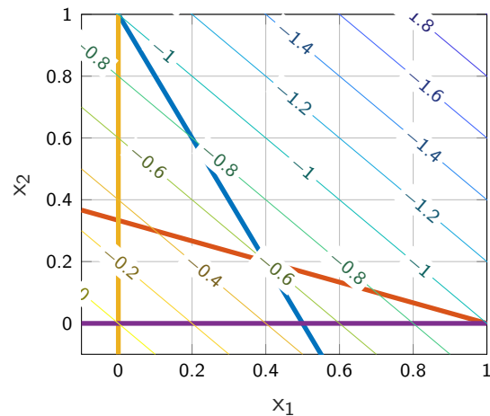
Abbildung 1: Höhenlinien und optimale Punkte für die verschiedenen Kostenfunktionen.
